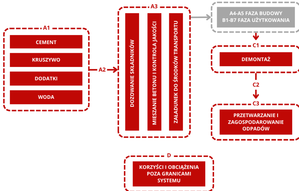
Rysunek 5.1: Granice systemu wykorzystane do charakterystyki środowiskowej betonu towarowego
